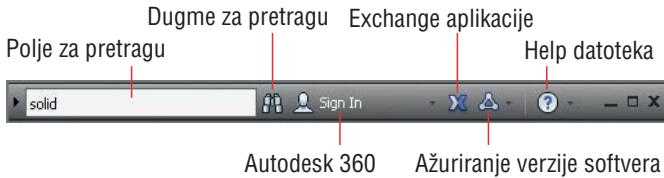
SLIKA 1.15 InfoCenter
